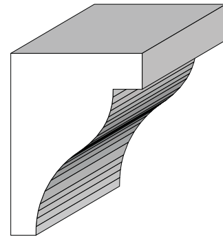
BA 679 1" x 1-3/8"
